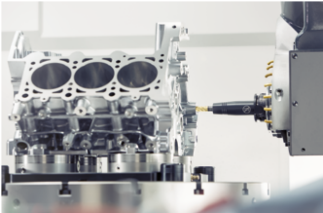
Bearbetning av cylinderhuvud med Tendo Slim 4ax
